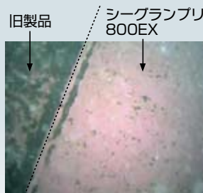
就航後 10 ヶ月での水中調査
