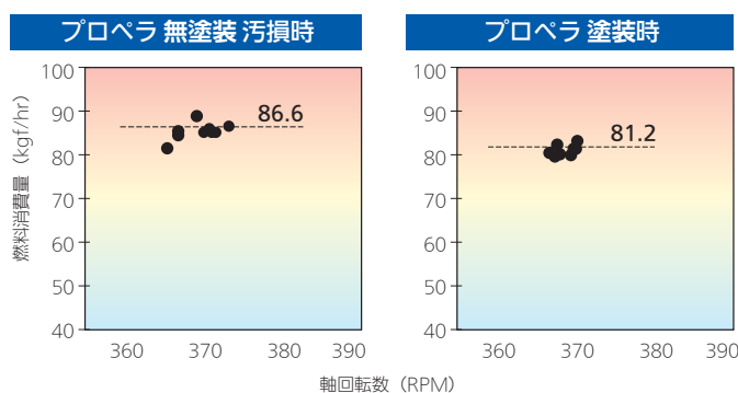
プロペラ 無塗装時と塗装時の機関性能の比較
